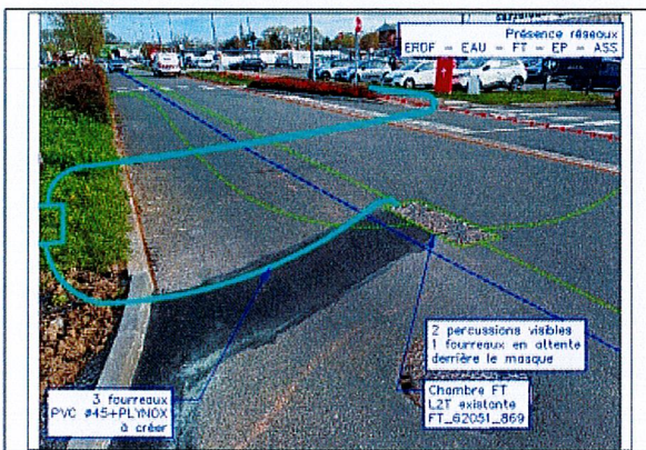
Chambre à percuter FT_62051_869
